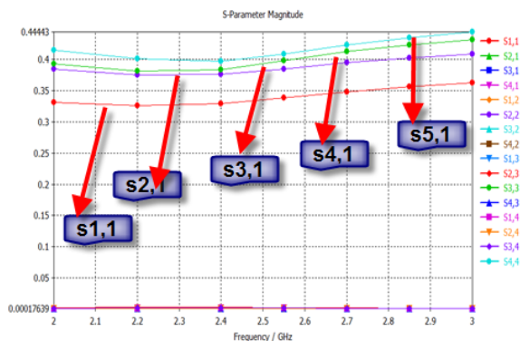
Fig.7 linear S-parameter of design antenna
