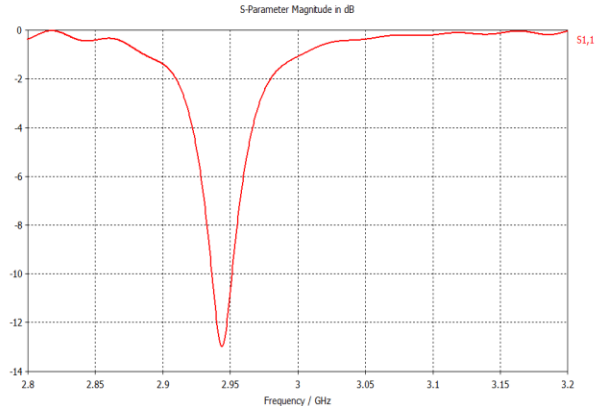
Fig. 2. S parameter magnitude
