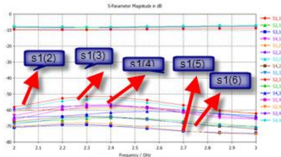
Fig.8 S - parameter of RFID antenna dB
